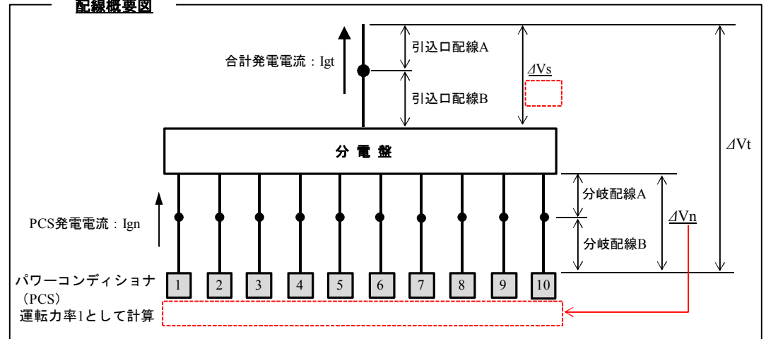
配線概要図
