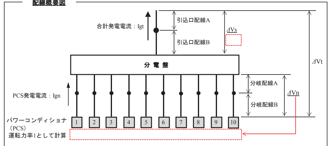
配線概要図
