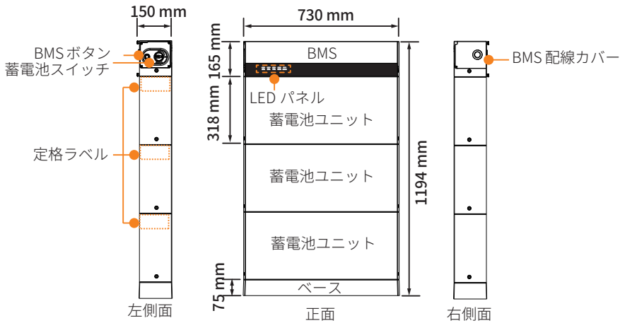
図 2-5 蓄電池の外観
