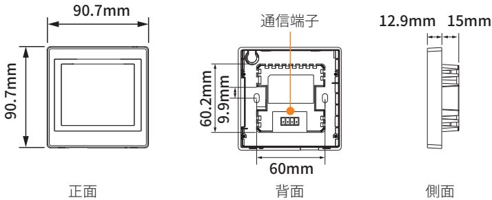
図 2-6 室内リモコンの外観
