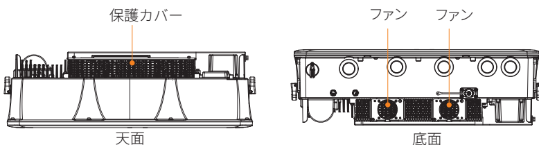
図 2-4 J1-Hybrid 9.9kW-2外観
