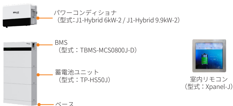
図 2-1 システム構成例
