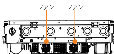
J1-Hybrid 9.9kW-2 底面
