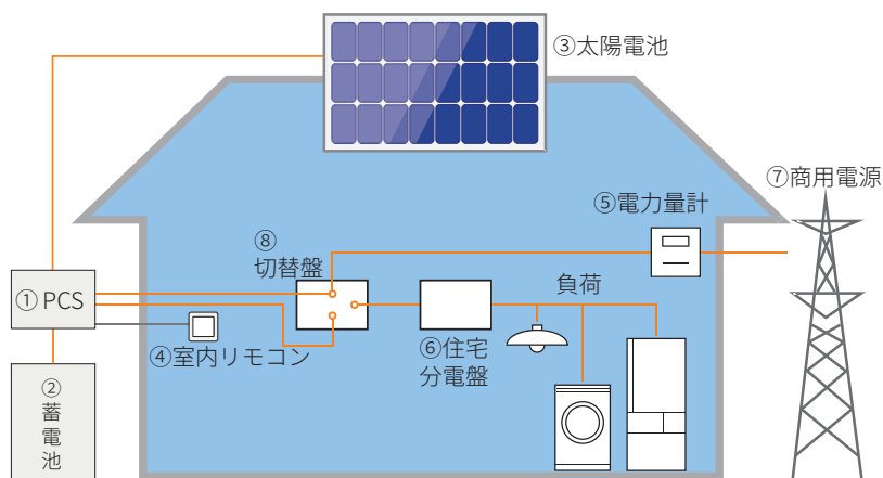
図 2-2 蓄電システム構成例
