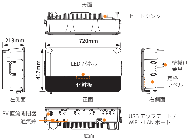
図 2-3 J1-Hybrid 6kW-2外観
