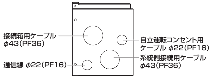
配線カバーへの穴開け箇所 (PF 管呼びで表記)
