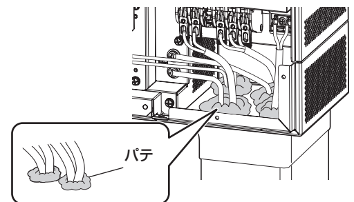
シーリング処理 (全周)
