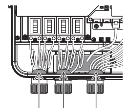
電線管(PF管)先端の隙間にパテ埋め
