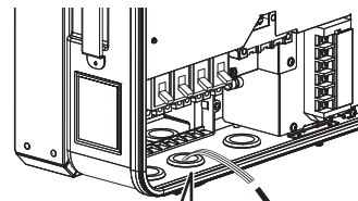
コーキング （変性シリコーン材）
