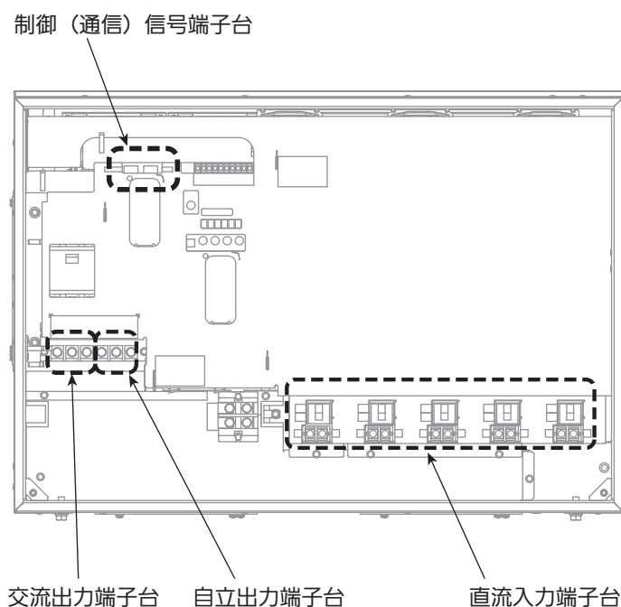
パワーコンディショナ内部図
