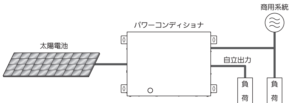
パワーコンディショナ構成図
