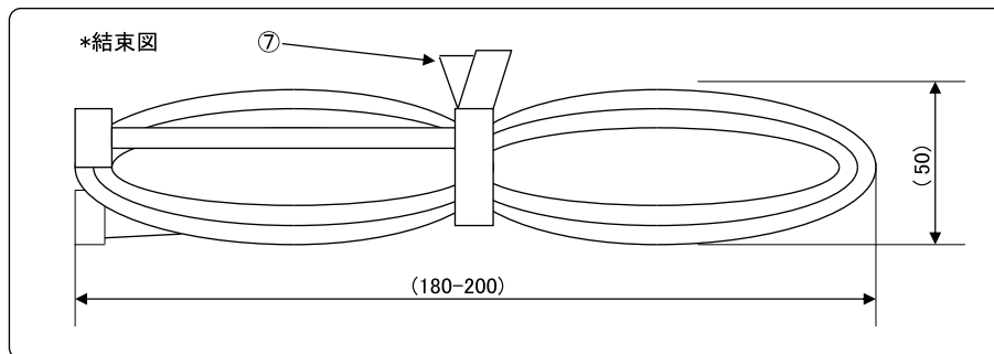
配線表
