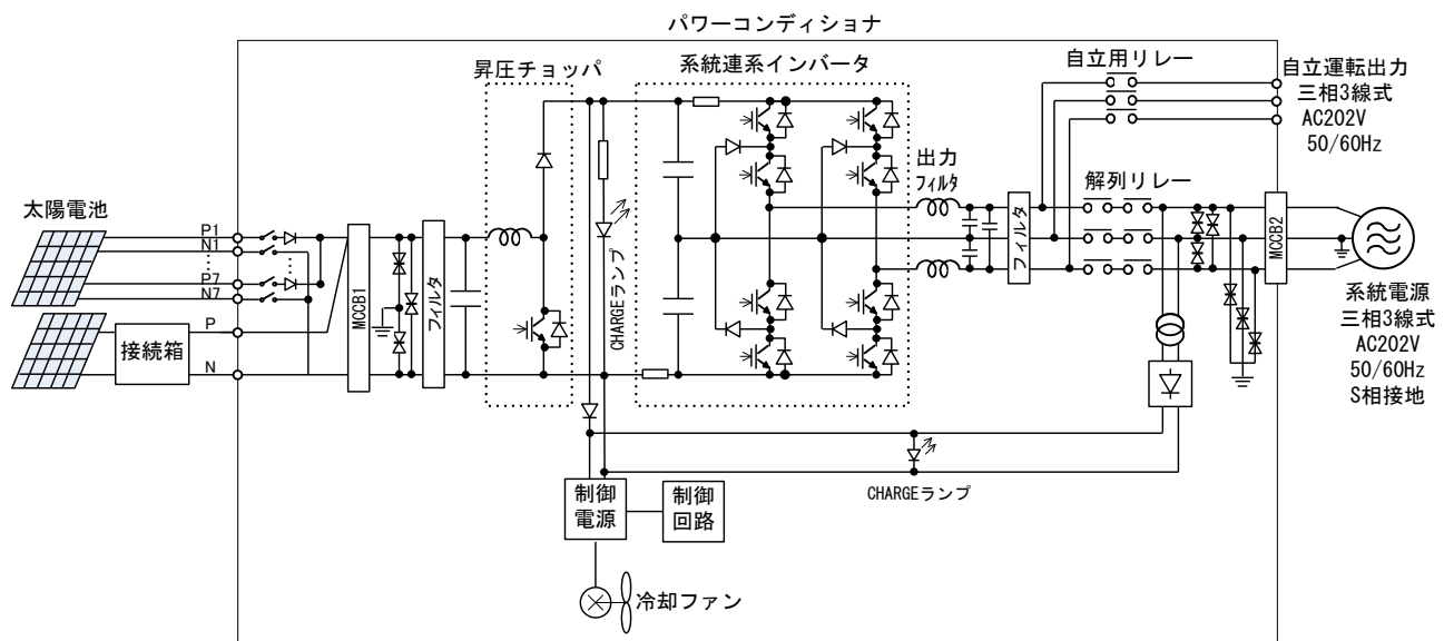
図2 主回路構成
